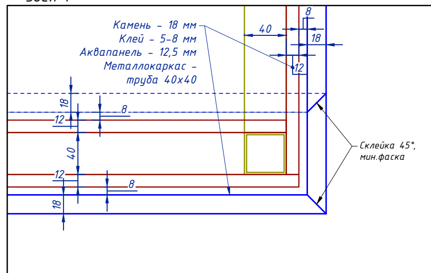
Узел 1
