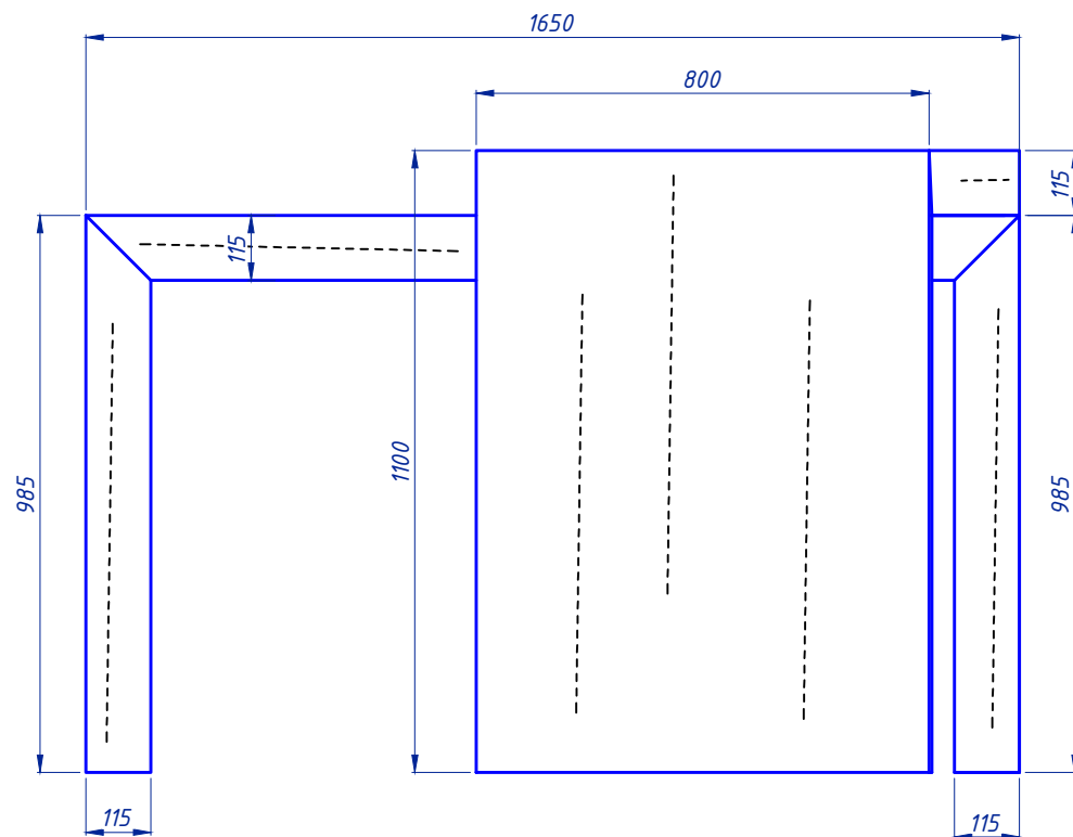
Вид 3
