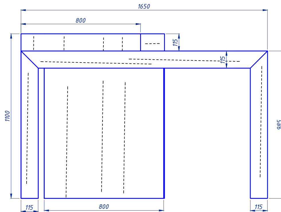
Вид 2
